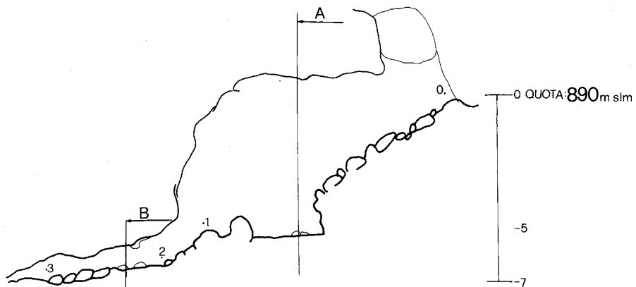
SEZIONE LONGITUDINALE
